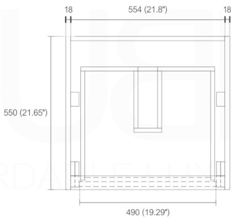
. TOP ELEVATION
